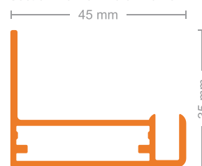
Profilato per intelaiatura Micron Section view of Micron frame
