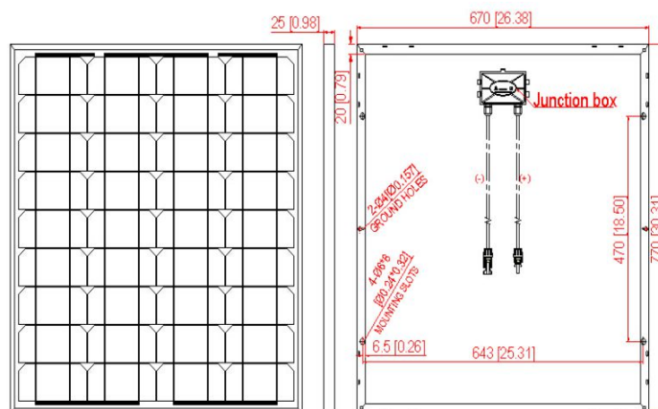
Module Diagram
