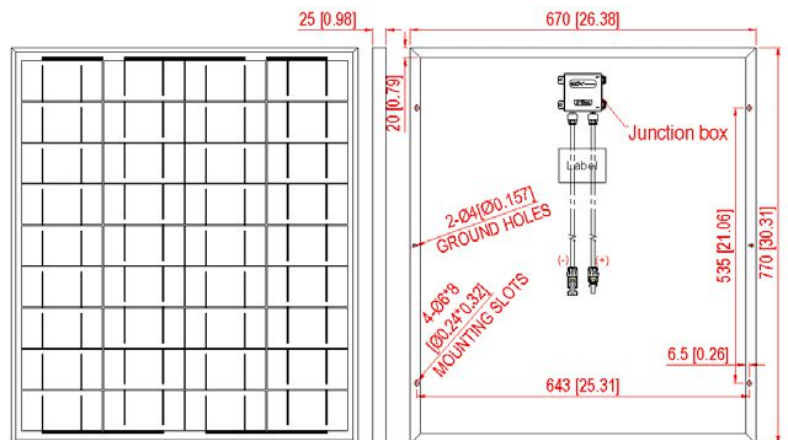
Module Diagram
