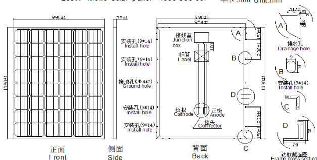
200W单晶硅太阳能电池板 (1330*990*35) 200W Mono solar panel (1330*990*35) 单位:mm Unit:mm
