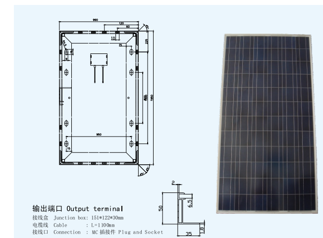
YHM290-30P
