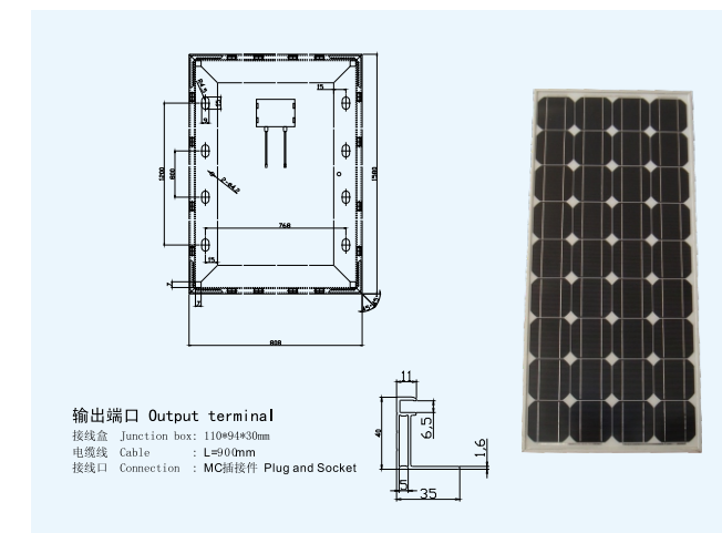
YHM190-36M
