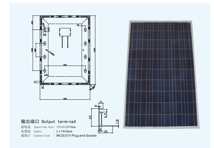
YHM240-30P
